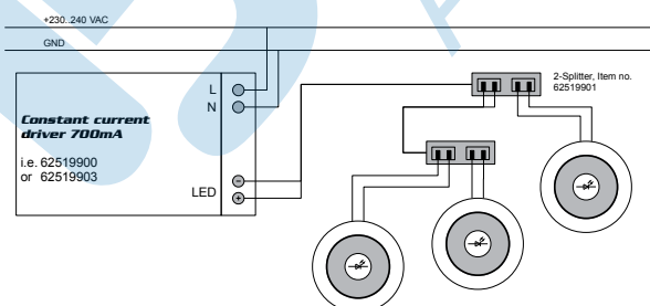
Anschlusskizze Pescara CC
